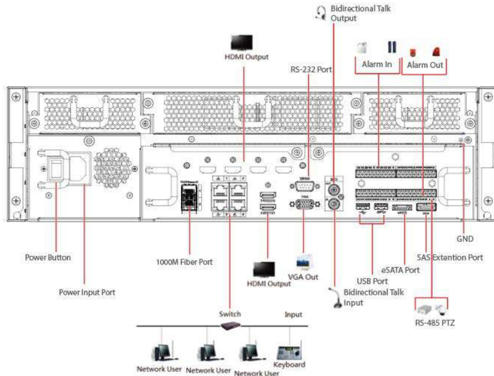
Figura 3-62 Conexiune tipică
