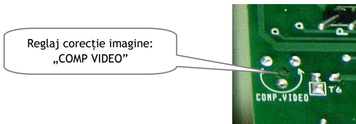
Fig. 23 Detaliu reglaj compensare, pe placa electronică P4S.V(A)91G
